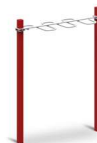
12091 Рукоход-змейка. Гефест 07 Материалы: сталь Длина: 2120 мм Высота: 2600 мм Ширина: 630 мм
